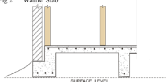
Fig 2 Waffle Slab
